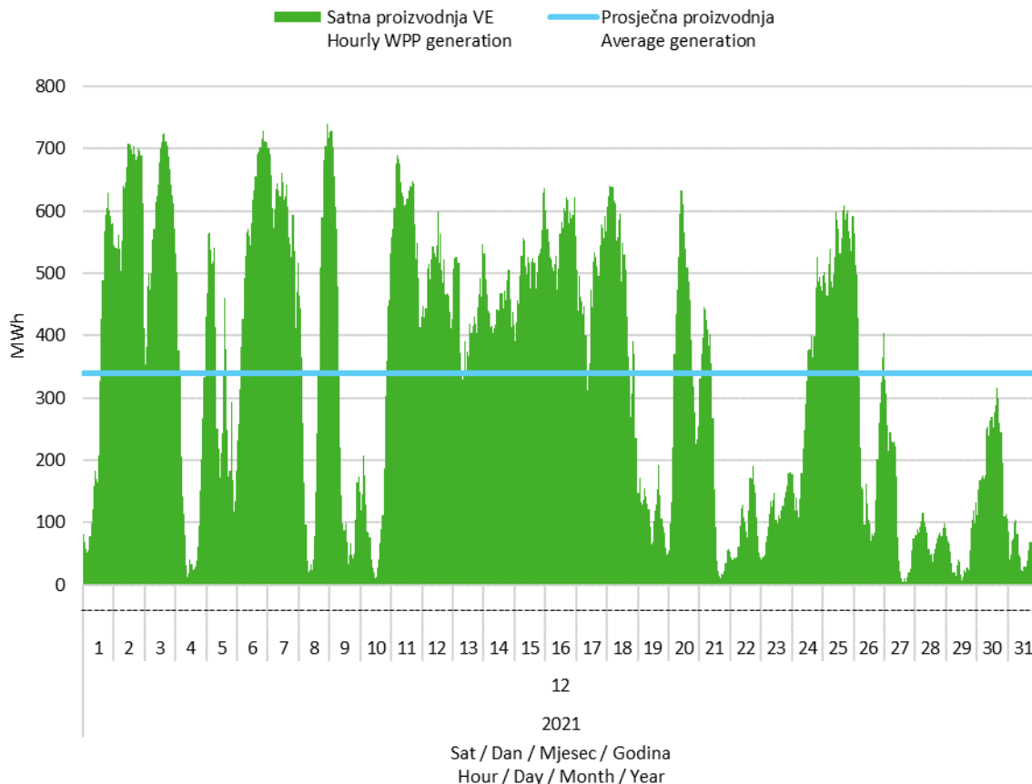
Slika 2 Satna proizvodnja svih vjetroelektrana u prosincu 2021. godine
