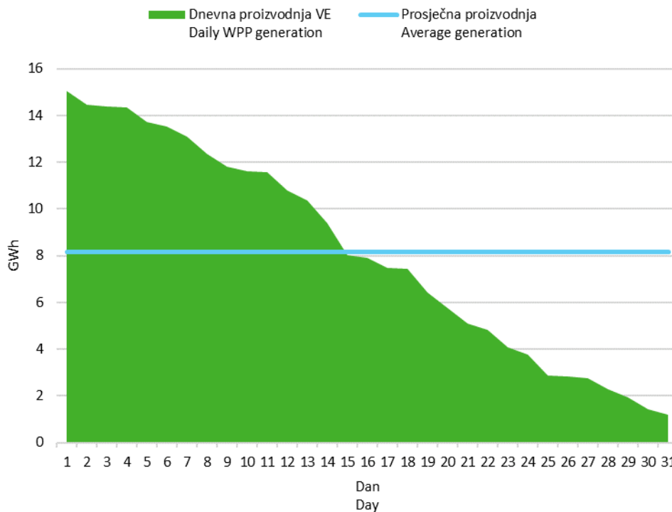
Slika 6 Krivulja trajanja dnevne proizvodnje vjetroelektrana u prosincu 2021. godine
