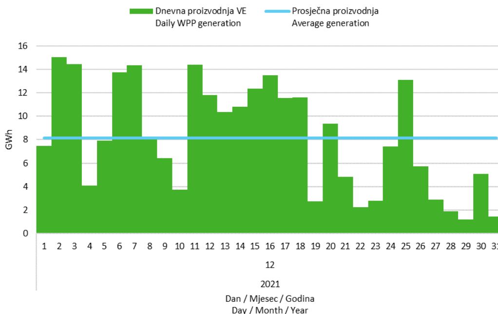
Slika 5 Dnevna proizvodnja svih vjetroelektrana u prosincu 2021. godine
