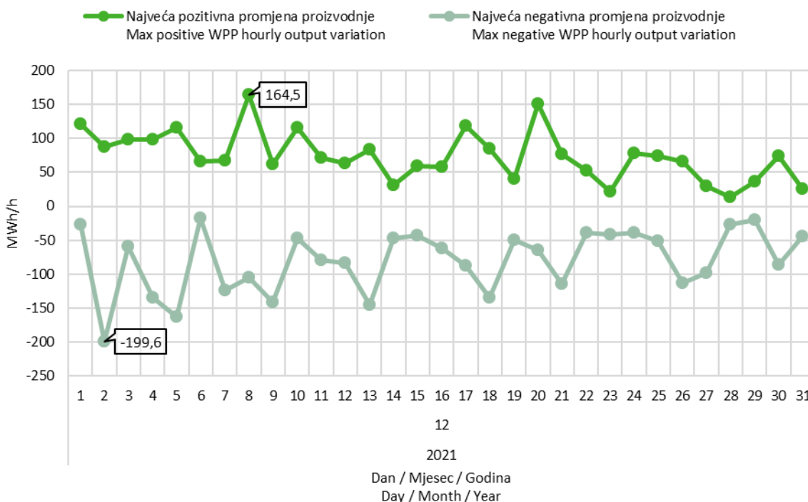
Slika 9 Maksimalna pozitivna i maksimalna negativna promjena satne proizvodnje VE u prosincu 2021. godine
