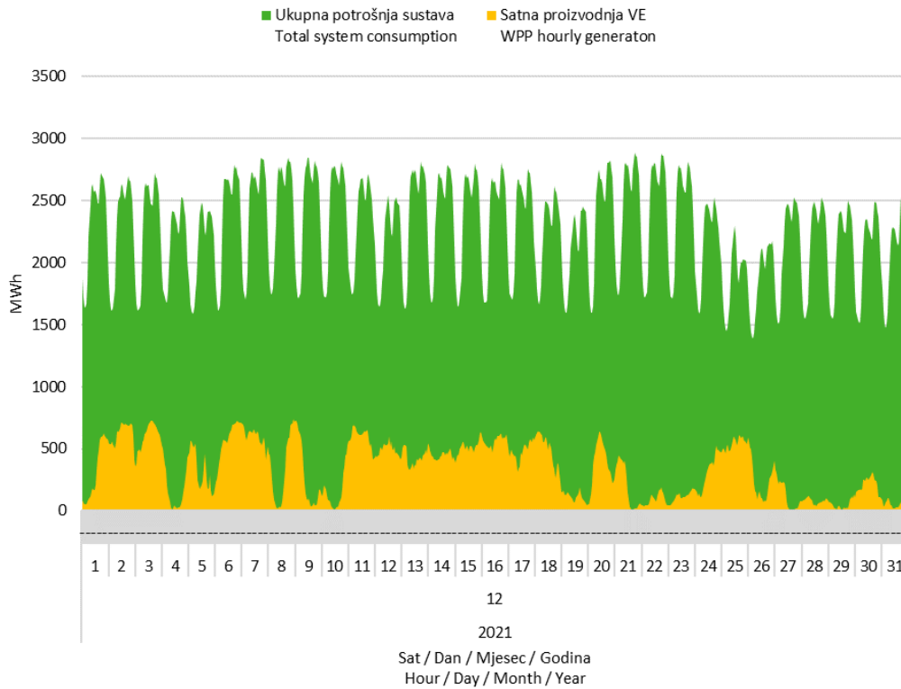
Slika 7 Usporedba satnog dijagrama opterećenja sustava i proizvodnje vjetroelektrana u prosincu 2021. godine
