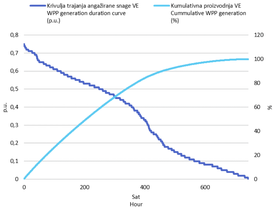
Slika 3 Krivulja trajanja angažirane snage svih VE i kumulativna proizvodnja VE u prosincu 2021. godine u jediničnim vrijednostima
