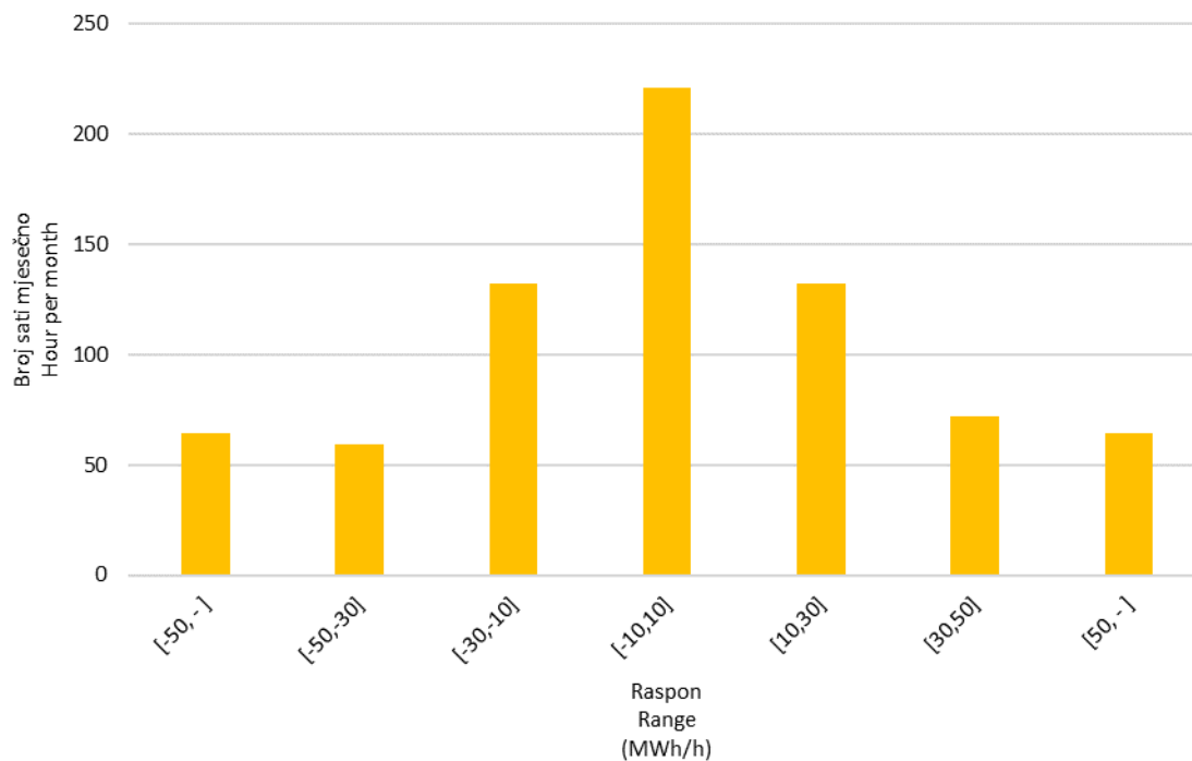
Slika 10 Statistička raspodjela satnih promjena proizvodnje VE u prosincu 2021. godine Figure 10 Statistical distribution of WPP hourly output variations in December 2021
