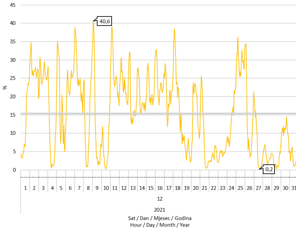
Slika 8 Udio proizvodnje vjetroelektrana u pokrivanju satnog opterećenja elektroenergetskog sustava u prosincu 2021. godine
